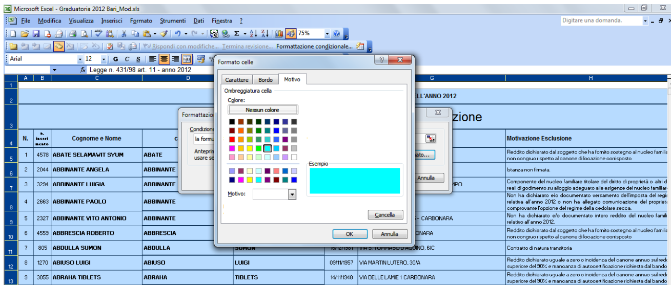
Figura 38 Scelta colore
