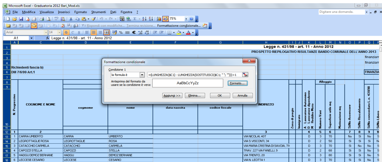
Figura 7 Digitazione formula
