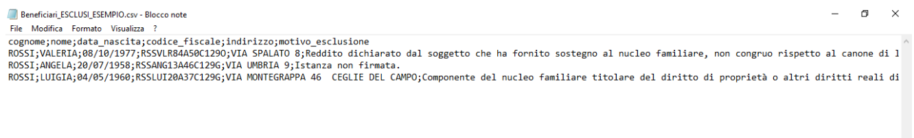
Figura 43 Aggiunta intestazione
