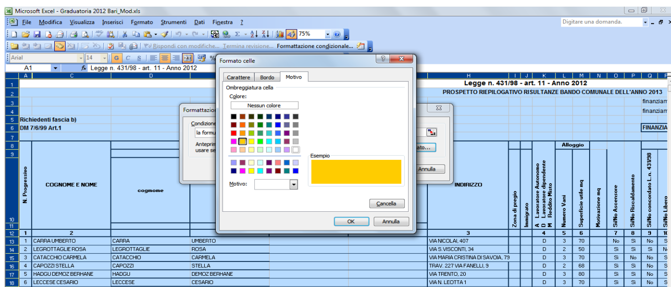
Figura 23 Scelta colore
