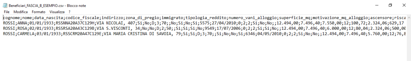
Figura 30 Aggiunta intestazione
