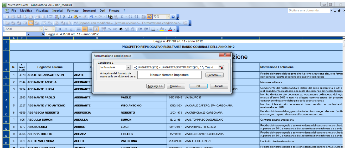
Figura 37 Digitazione formula
